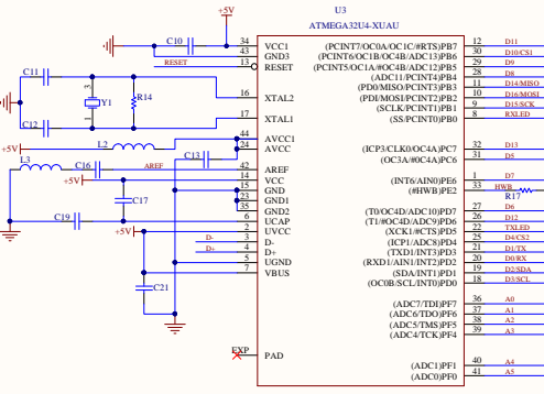
Input Unit
