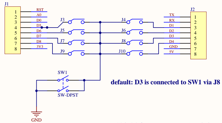
Button Shield for WeMos D1 Mini
