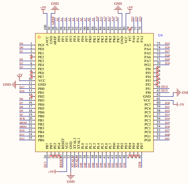
MCU Unit
